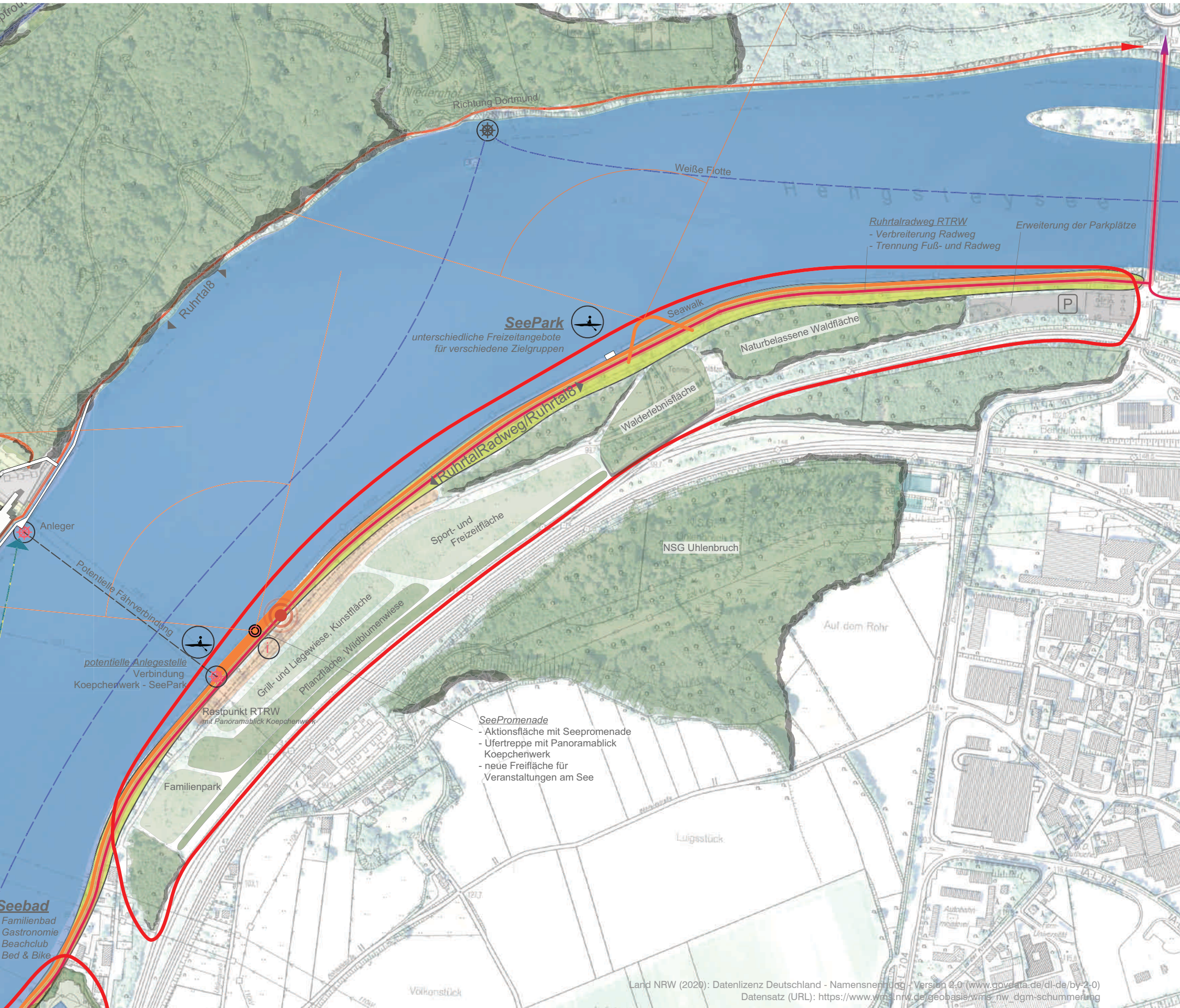
Abb. 59 Entwicklungsskizze SeePark Hengstey (Qu.: DTP auf Grundlage Land NRW)
