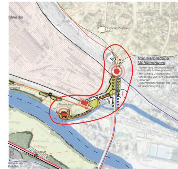
Abb. 37 Entwicklungsskizze Ruhrfenster Mühlengraben (Qu.: DTP auf Grundlage Land NRW)
